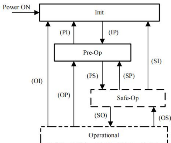
图 5-2 从站状态机示意图
